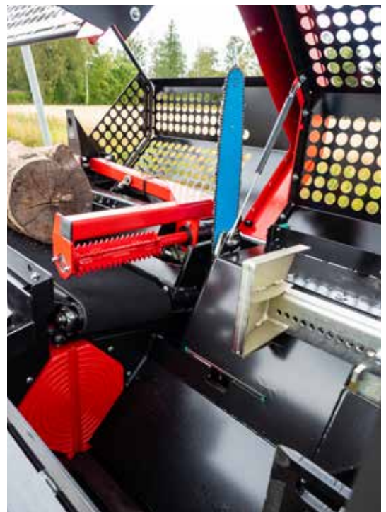
Upínání kulatiny s hydraulickým hnacím válečkem zajišťuje efektivní podávání kulatiny.
